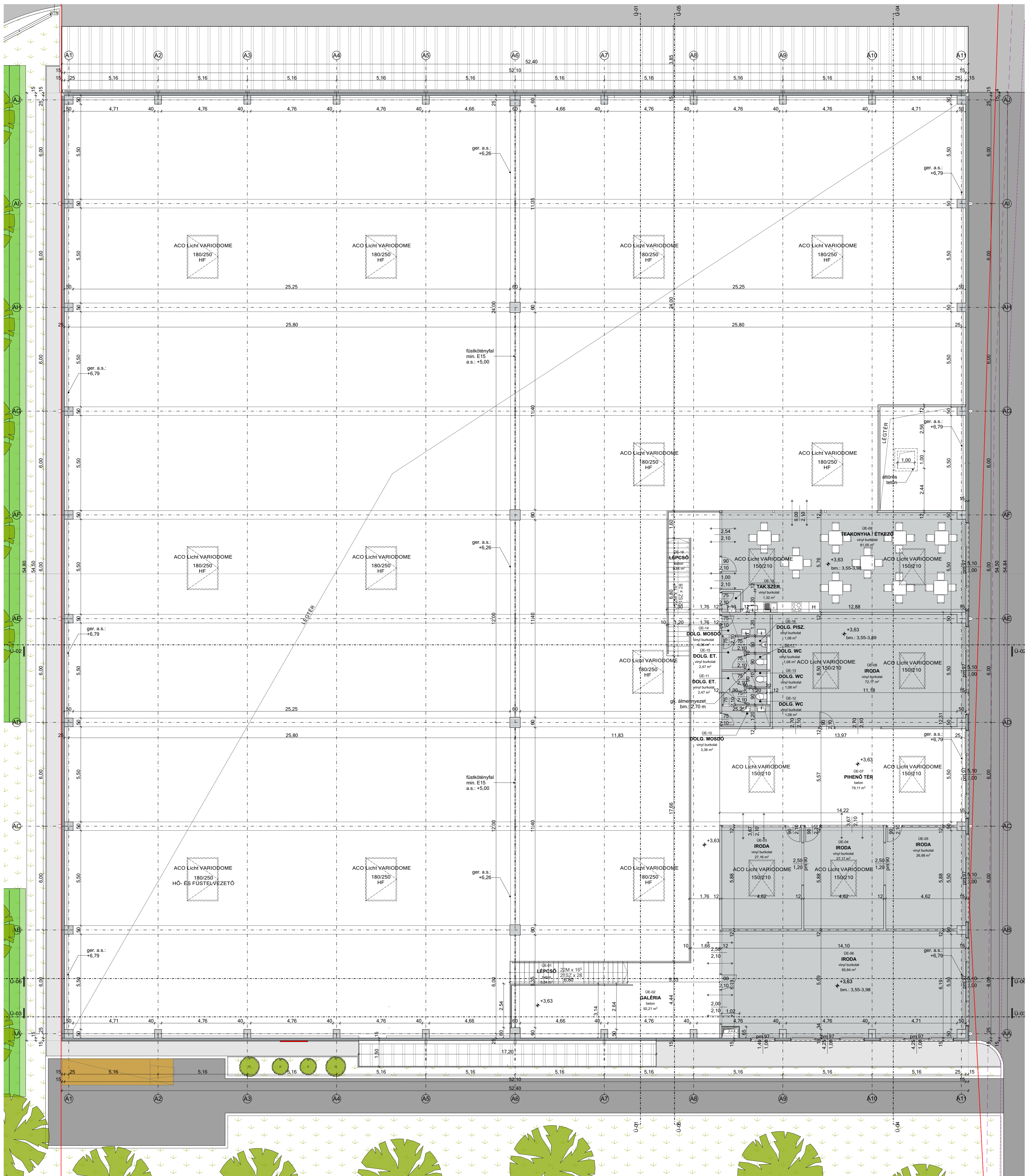
EMELET ALAPRAJZ - ÜZEMCSARNOK
