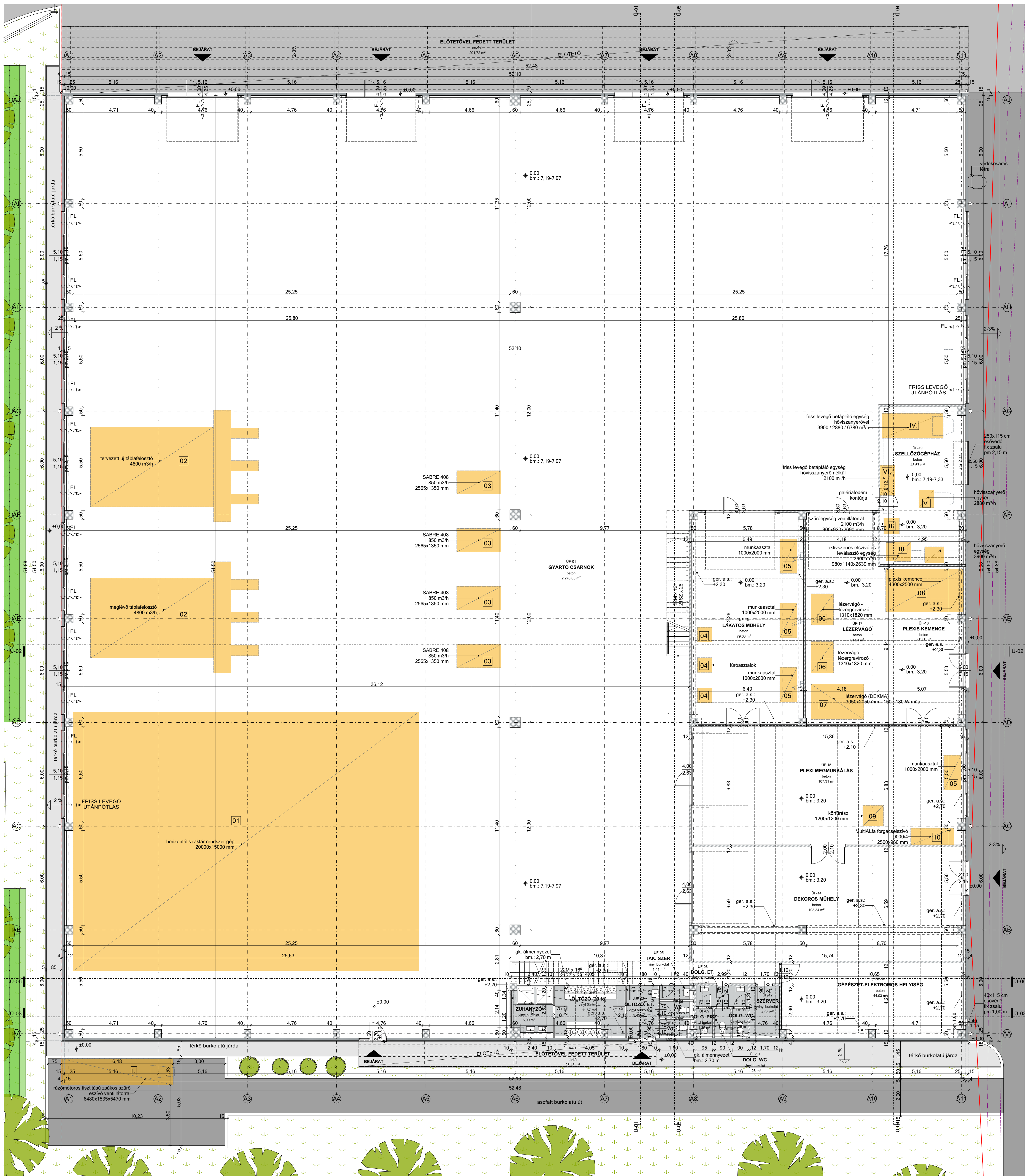
FÖLDSZINT ALAPRAJZ - ÜZEMCSARNOK
